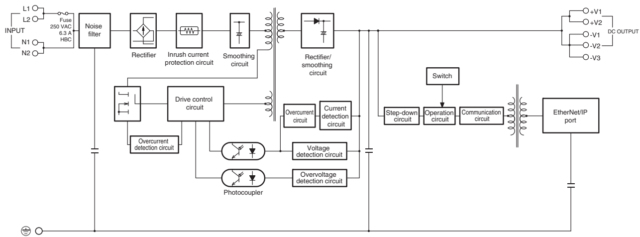
S8VK-X09024-EIP
